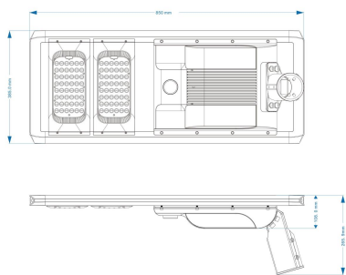
FX-40W
